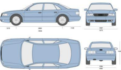
Audi A8 (2000)
