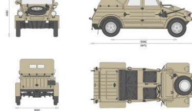
Volkswagen Kubelwagen (1945)
