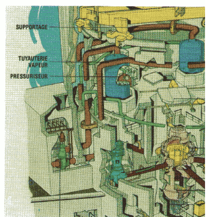
Vue intérieure d'une enceinte nucléaire ►
